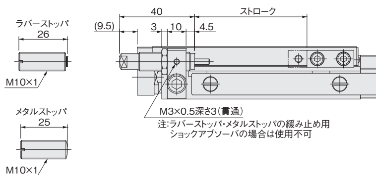
配管口方向-Lの場合
